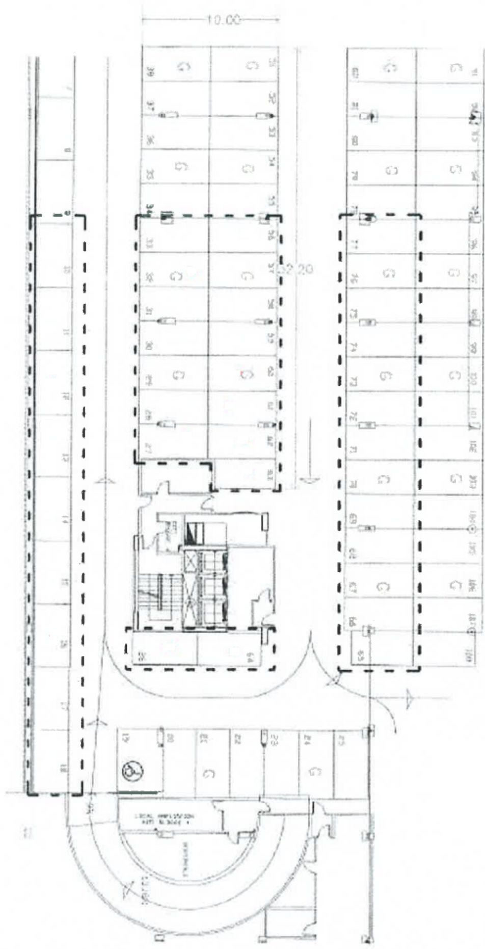
PLANTA SOTANO 1
